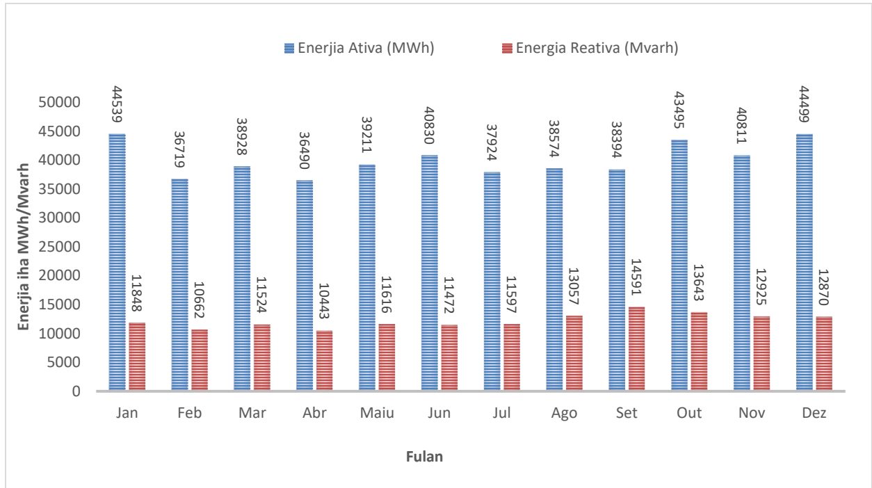
Figura 14 Komparasaun Enerjia Ativa vs Enerjia Reativa kada Fulan iha Tinan 2021
