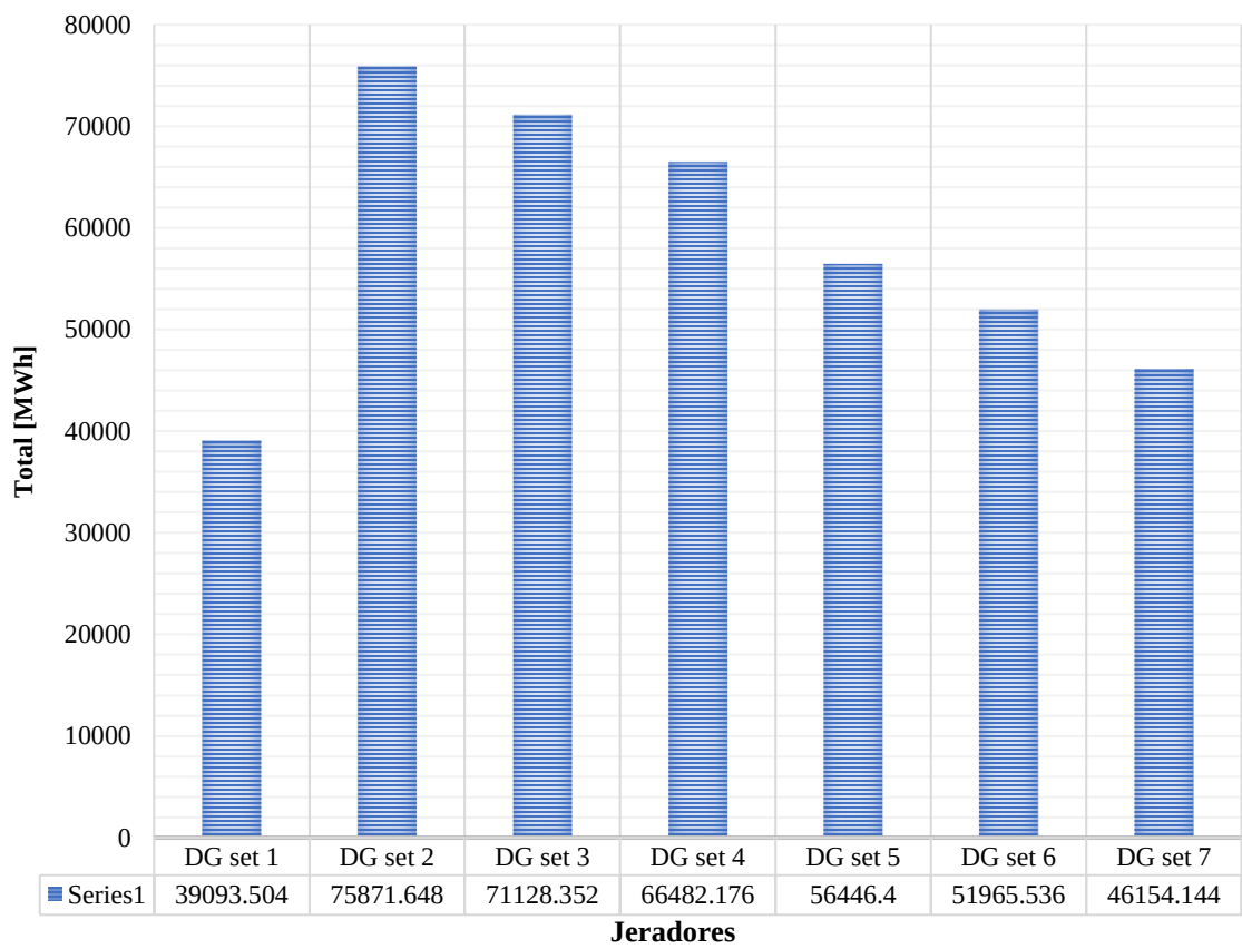
Figura 11 Gráfiku Meter Reading ba Kada Jeradór iha Sentráel Elétrika Hera
